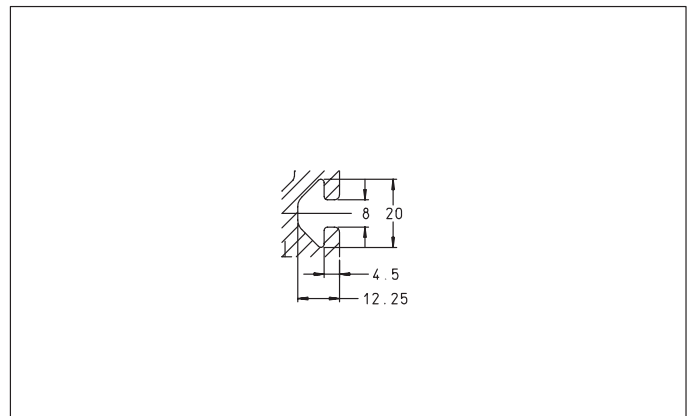
T-grooves
