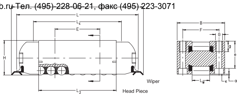
RUS 19 069 to RUS 38 206
