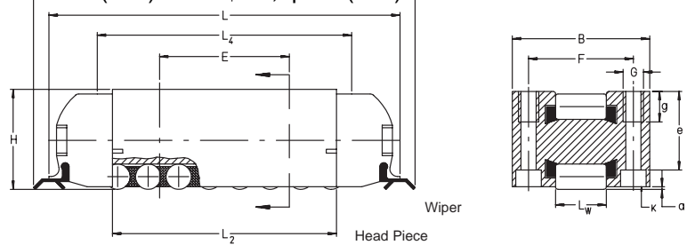
RUS 19 069 to RUS 38 206
