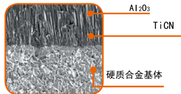
Al 2 O 3
